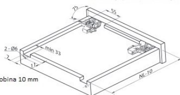
Dimenzije predala in vrtnanje
