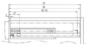
Standardni predal, LTmin=NL+3 LT-notranja odprtina omarice
