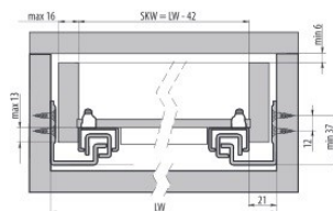
SKW-notranje mere predala
