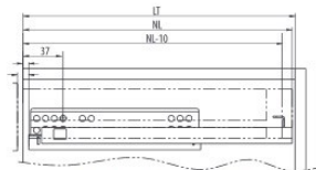
Standardni predal, LTmin=NL+3 LT-notranja odprtina omarice
