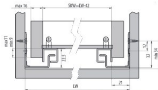
SKW-notranje mere predala
